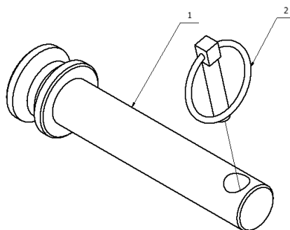
Rys. 70. Sworzeń zaczepowy górny kompletny Ø32mm.
