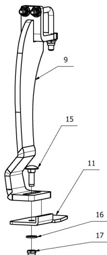
Rys. 57. Wał gumowy \varnothing 500\text{mm} – skrobak.
