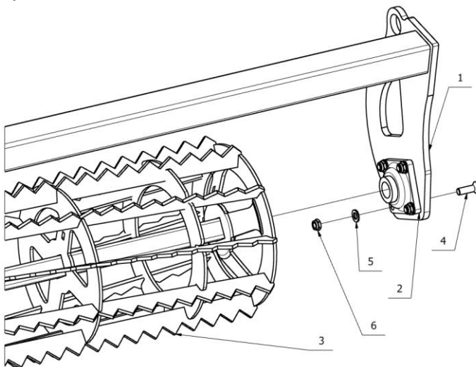
Rys. 18. Wał strunowy Ø420mm.
