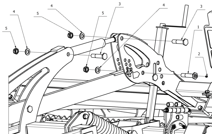
Rys. 4. Mocowanie ramienia regulacyjnego wału.
