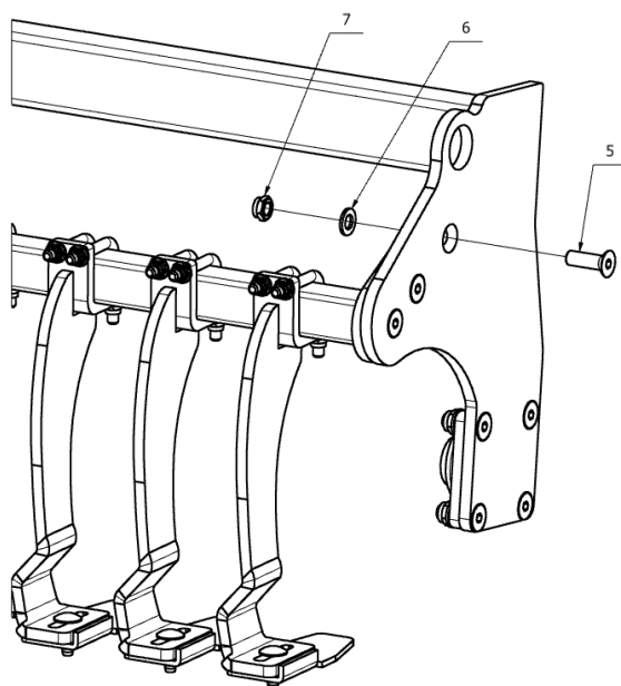
Rys. 55. Wał gumowy \varnothing 500\text{mm} – mocowanie belki ze skrobakiem w części bocznej.
