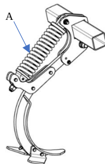
Rysunek 13. Ząb maszyny z zabezpieczeniem sprężynowym.
