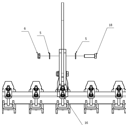
Rys. 23. Mocowanie podpory dolnej wspornika środkowego.
