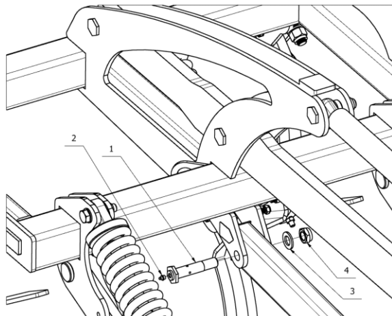
Rys. 7. Mocowanie belki talerzowej
