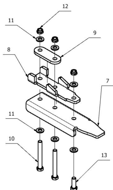
Rys. 31. Skrobak.
