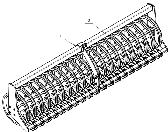
Rys. 37. Wał ceownikowy Ø520mm.
