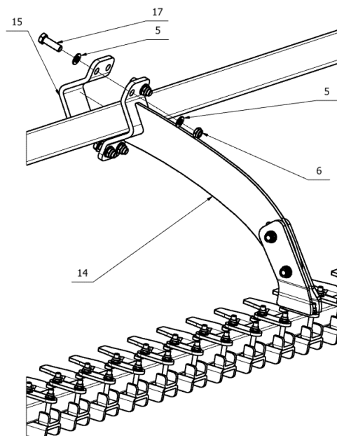
Rys. 45. Wał teownikowy \varnothing 600\text{mm} – górne mocowanie wspornika środkowego.
