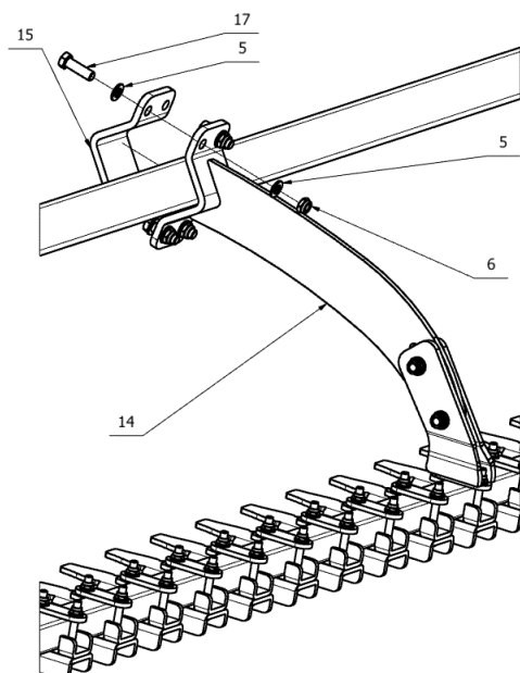
Rys. 40. Wał ceownikowy Ø520mm – górne mocowanie wspornika środkowego.
