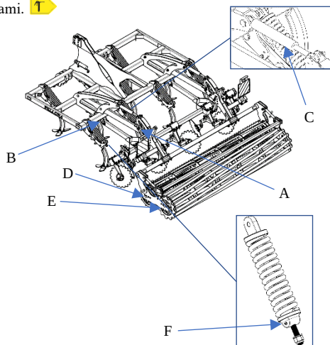
Rysunek 16. Punkty smarowania.
