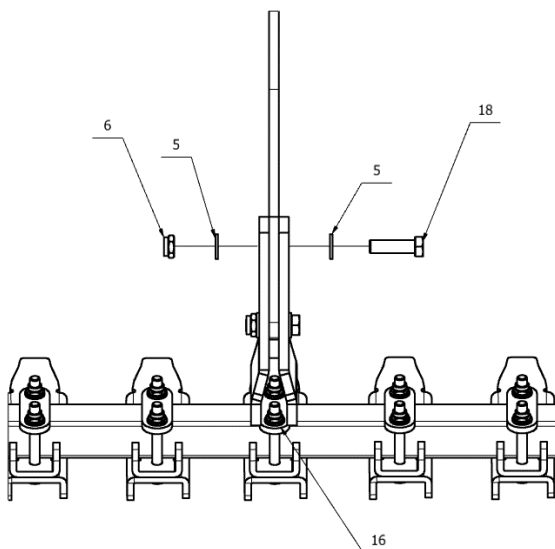
Rys. 28. Mocowanie podpory dolnej wspornika środkowego.
