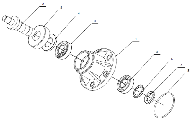
Rys. 12. Piasta.
