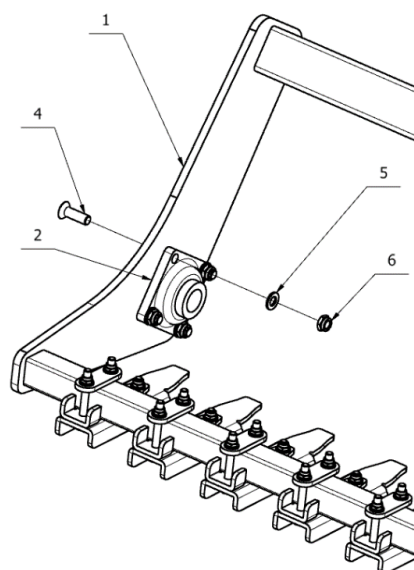
Rys. 25. Wał daszkowy Ø600mm - mocowanie łożyska.
