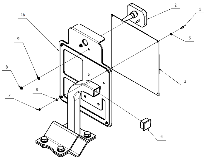
Rys. 74. Tablica oświetleniowa prawa.
