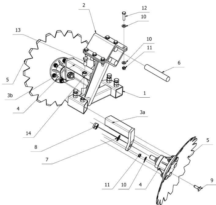
Rys. 10. Zespół talerzy belki niwelującej.
