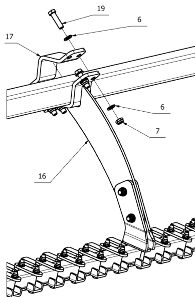
Rys. 51. Wał dyskowy Ø600mm – górne mocowanie wspornika środkowego.
