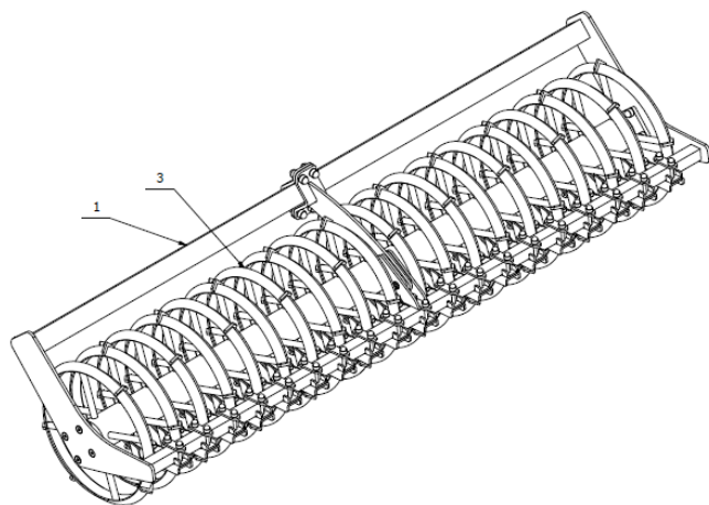
Rys. 19. Wał daszkowy Ø500mm.
