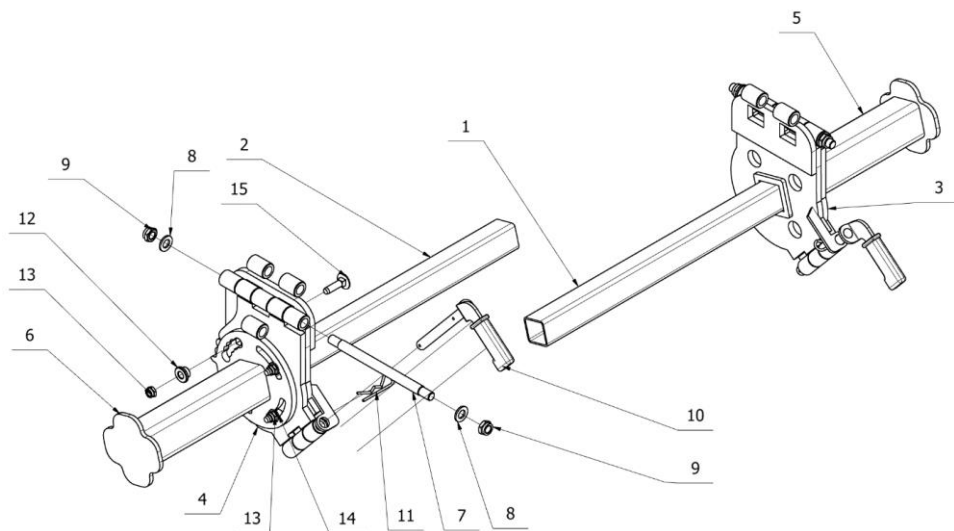
Rys. 13. Zawiasy.
