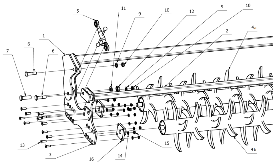
Rys. 68. Wał tandem mulczujący.
