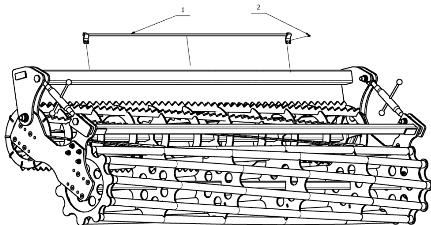
Rys. 76. Pręt mocowania oświetlenia.
