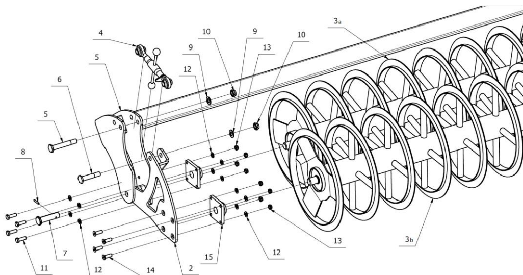
Rys. 67. Wał tandem teownikowy Ø600mm.
