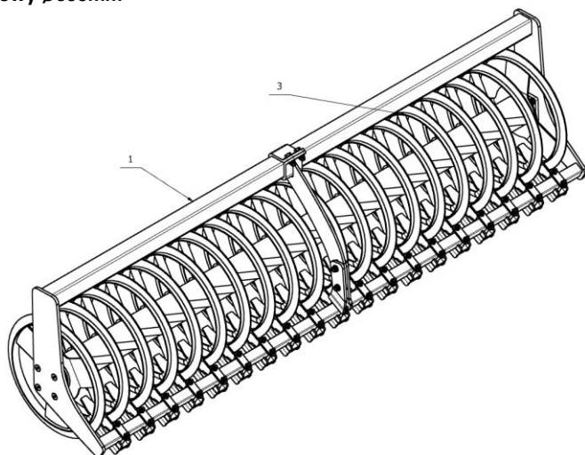
Rys. 42. Wał teownikowy Ø600mm.
