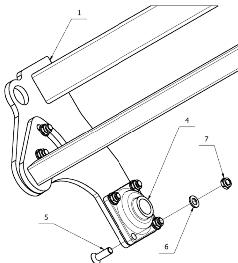
Rys. 54. Wał gumowy \varnothing 500\text{mm} – mocowanie łożysk.
