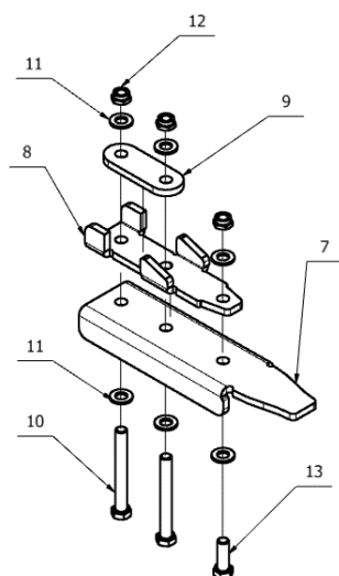
Rys. 26. Skrobak.
