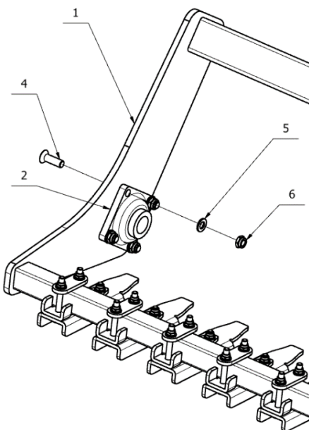
Rys. 30. Wał daszkowy Plus Ø600mm na profilu - mocowanie łożyska.
