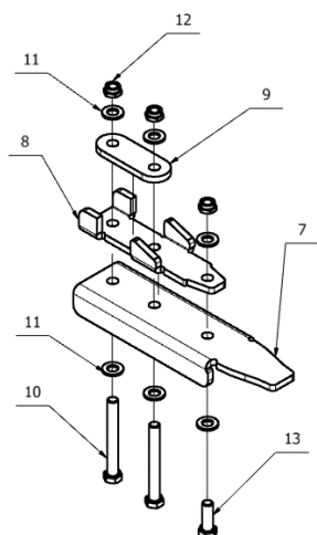
Rys. 39. Wał ceownikowy Ø520mm – skrobak.
