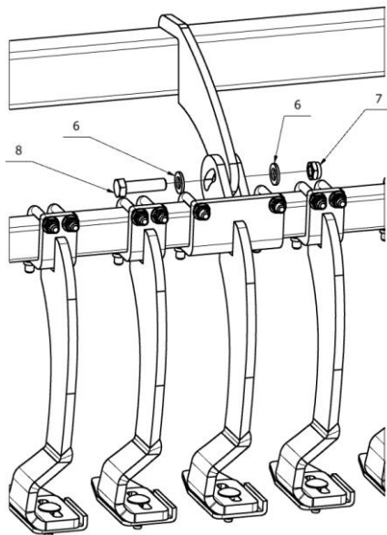
Rys. 56. Wał gumowy \varnothing 500\text{mm} – mocowanie belki ze skrobakiem w części środkowej.
