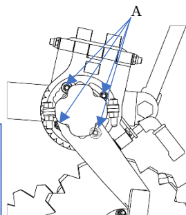
Rysunek 11. Ustawianie głębokości pracy skrajnego talerza.
