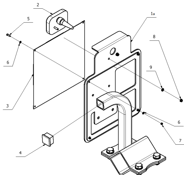
Rys. 74. Tablica oświetleniowa prawa.
