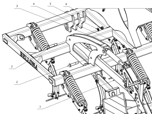
Rys. 3. Mocowanie głównego ramienia wału.
