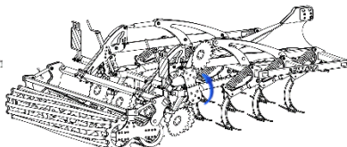
Rysunek 12. Składanie skrajnych talerzy do transportu.
