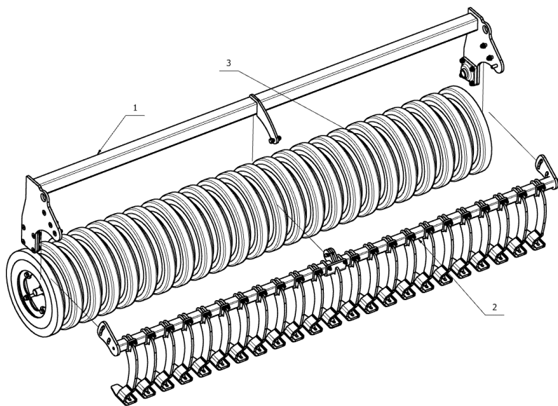
Rys. 53. Wał gumowy Ø500mm.
