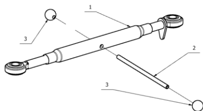
Rys. 6. Śruba regulacji głębokości roboczej.
