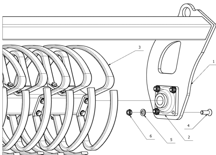
Rys. 35. Wał pierścieniowy \varnothing 500\text{mm} - mocowanie łożyska.
