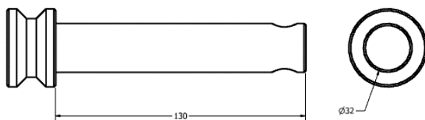
Rys. 70. Sworzeń zaczepowy górny kompletny Ø32mm.
