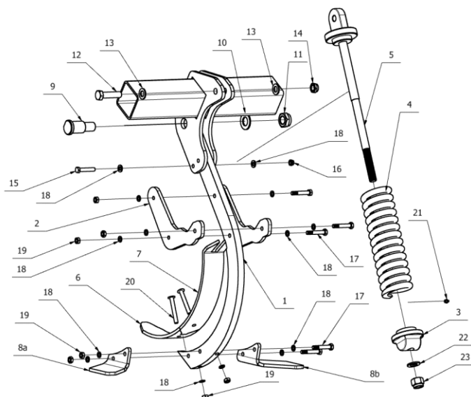
Rys. 2. Zespół grządzieli.
