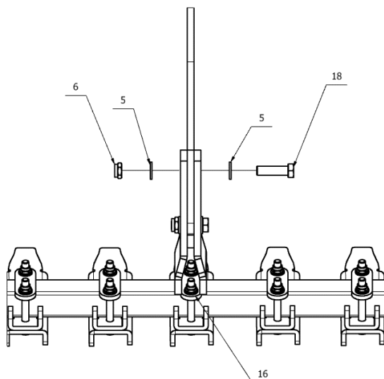
Rys. 46. Wał teownikowy Ø600mm – mocowanie podpory dolnej wspornika środkowego.
