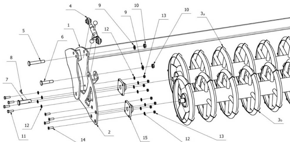
Rys. 64. Wał tandem daszkowy Ø500mm.
