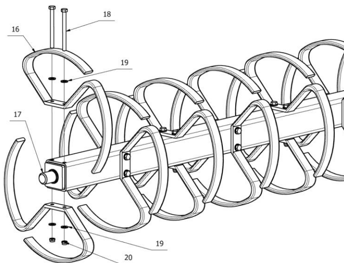
Rys. 63. Wał tandem pierścieniowy Ø500mm – mocowanie półpierścieni.
