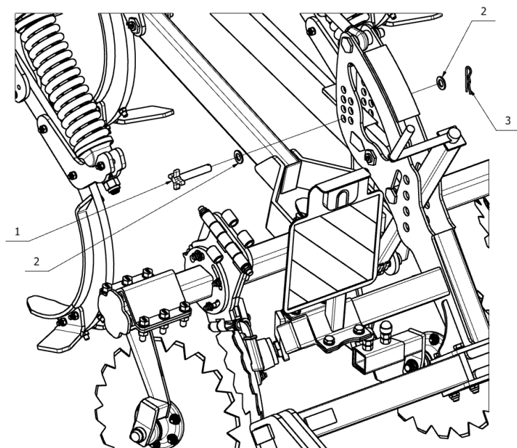
Rys. 15. Sworzeń docisku ramion.
