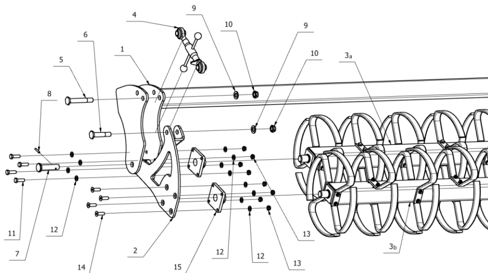
Rys. 62. Wał tandem pierścieniowy Ø500mm.
