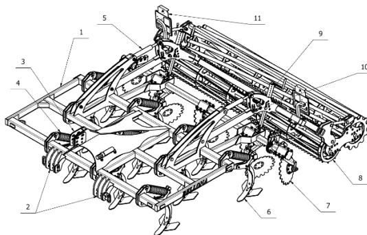
Rysunek 2. 1. Rama główna, 2. Zaczepy dolne, 3. Stojak z otworami, 4. Automatyczne zabezpieczenie przeciążeniowe zębów, 5. Hydrauliczna regulacja głębokości roboczej, 6. Grządziel, 7. Talerze niwelujące, 8. Wał tandem, 9. Regulacja głębokości pracy talerzy niwelujących, 10. Otwory blokujące ramiona wałów, 11. Światła.
