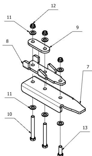
Rys. 44. Wał teownikowy \varnothing 600\text{mm} – skrobak.
