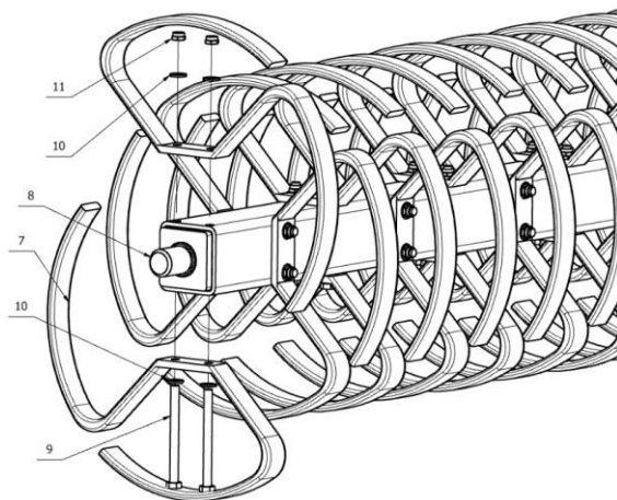
Rys. 36. Wał pierścieniowy Ø500mm - mocowanie pierścienia.
