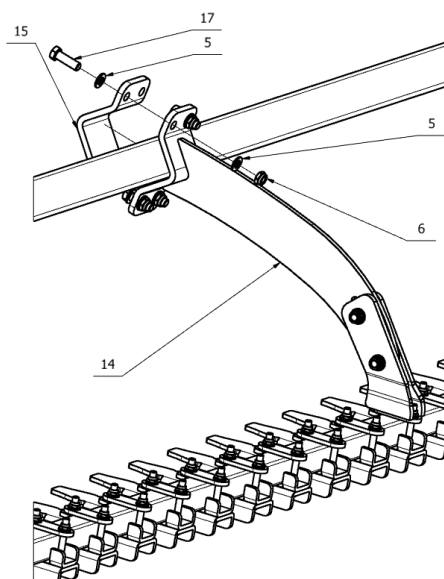
Rys. 22. Górne mocowanie wspornika środkowego.
