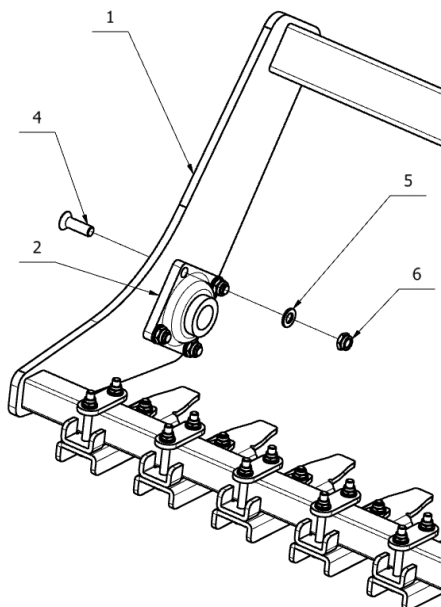
Rys. 43. Wał teownikowy Ø600mm - mocowanie łożyska.
