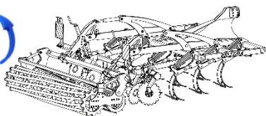
Rysunek 12. Składanie skrajnych talerzy do transportu.
