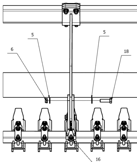
Rys. 33. Mocowanie podpory dolnej wspornika środkowego.
