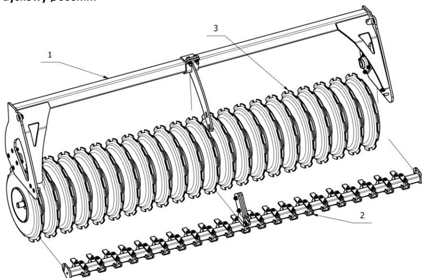
Rys. 47. Wał dyskowy Ø600mm.
