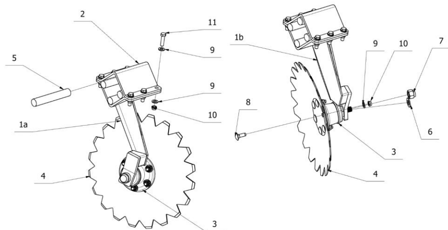
Rys. 11. Słupica pojedyncza.
