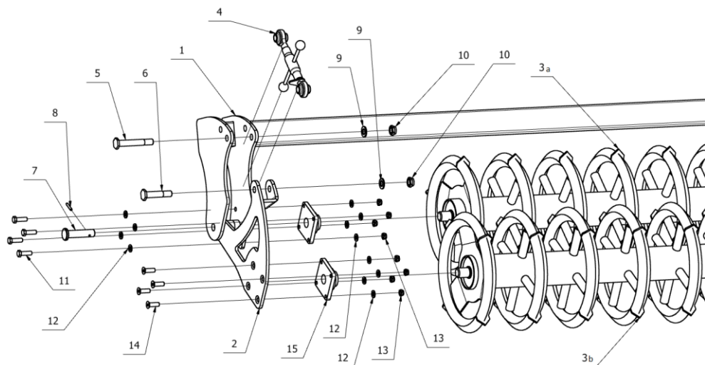
Rys. 65. Wał tandem daszkowy Plus Ø500mm.
