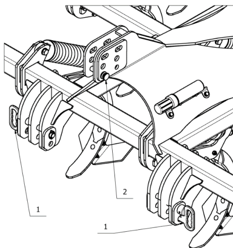
Rys. 69. Sworznie zaczepowe - mocowanie.
