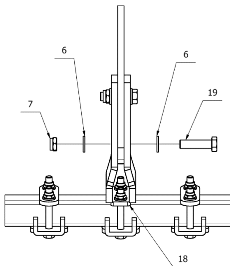
Rys. 52. Wał dyskowy Ø600mm – mocowanie podpory dolnej wspornika środkowego.
