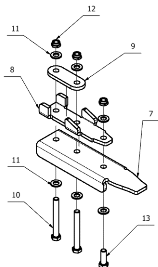
Rys. 21. Skrobak.
