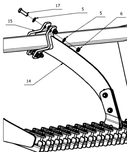
Rys. 32. Górne mocowanie wspornika środkowego.
