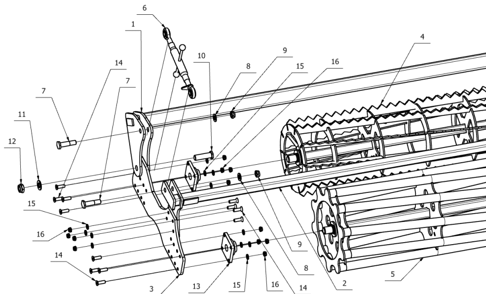
Rys. 60. Wał tandem rurowo (Ø500mm) – strunowy (Ø420mm).
