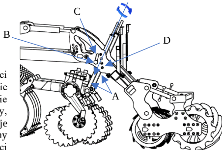
Rysunek 9. Regulacja głębokości pracy talerzy niwelujących.
