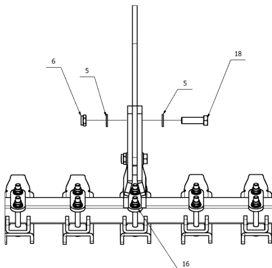
Rys. 41. Wał ceownikowy Ø520mm – mocowanie podpory dolnej wspornika środkowego.
