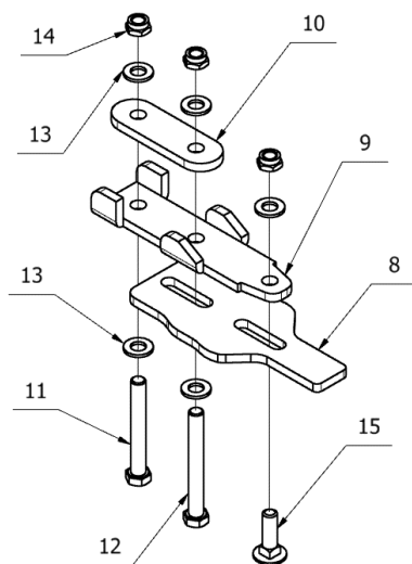
Rys. 50. Wał dyskowy \varnothing 600\text{mm} – skrobak.
