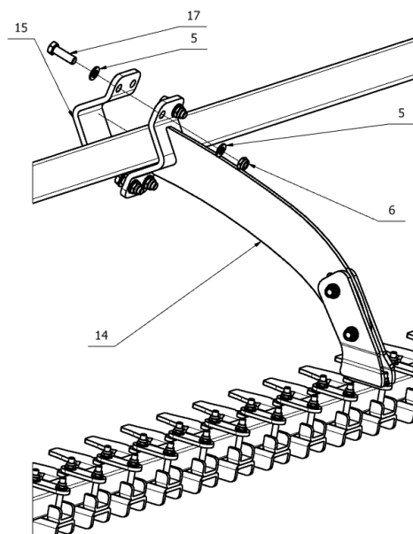
Rys. 27. Górne mocowanie wspornika środkowego.
