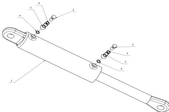
Rys. 5. Siłownik ramienia wału.
