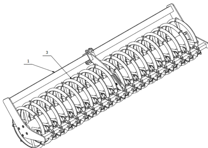
Rys. 24. Wał daszkowy Ø600mm.
