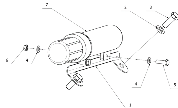
Rys. 79. Bidon na instrukcję.
