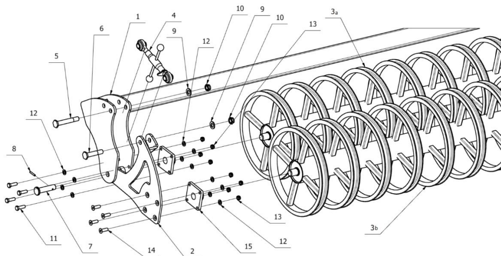
Rys. 66. Wał tandem ceownikowy Ø520mm.
