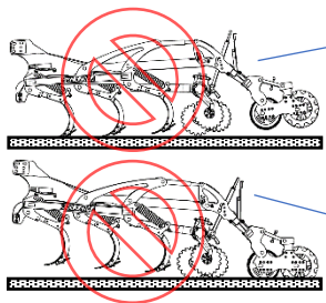
Rysunek 8. Regulacja ustawienia maszyny.
