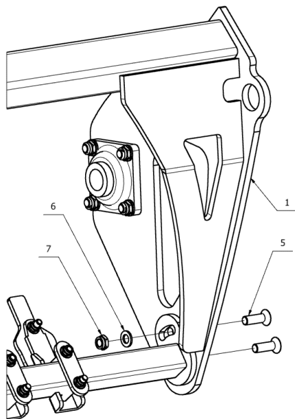
Rys. 49. Wał dyskowy \varnothing 600\text{mm} – mocowanie belki ze skrobakiem.
