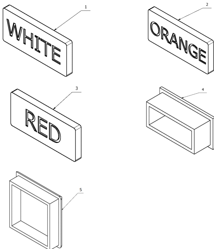
Rys. 87. Inne elementy.
