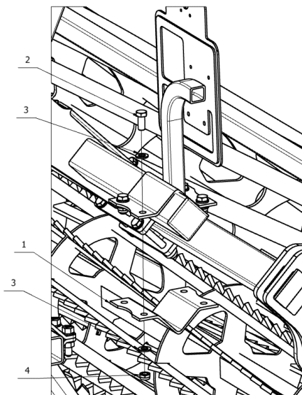
Rys. 73. Mocowanie oświetlenia na belce.
