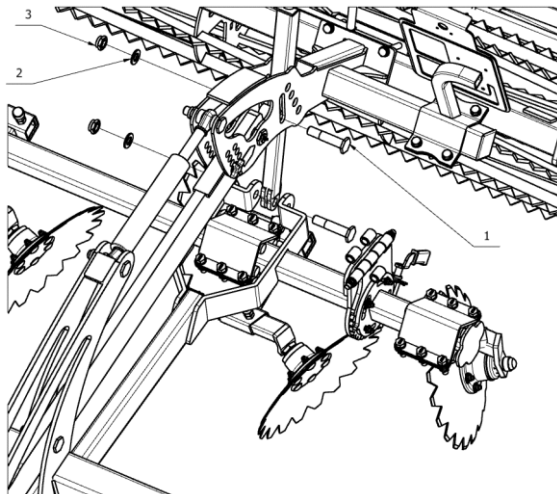
Rys. 8. Mocowanie śruby teleskopowej.
