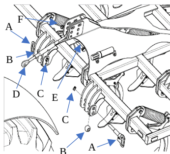
Rysunek 5. Podpinanie maszyny do ciągnika.
