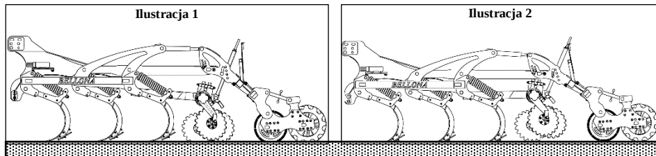
Rysunek 10. Różne ustawienia talerzy niwelujących. Ilustracja 1 - Praca głęboka, Ilustracja 2 - Praca płytka.
