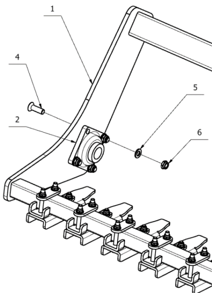
Rys. 20. Wał daszkowy Ø500mm - mocowanie łózyska.
