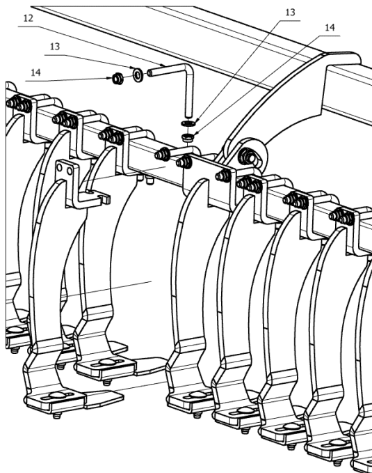
Rys. 59. Wał gumowy Ø500mm – mocowanie skrobaka na belce.
