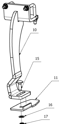
Rys. 58. Wał gumowy \varnothing 500\text{mm} – skrobak środkowy.
