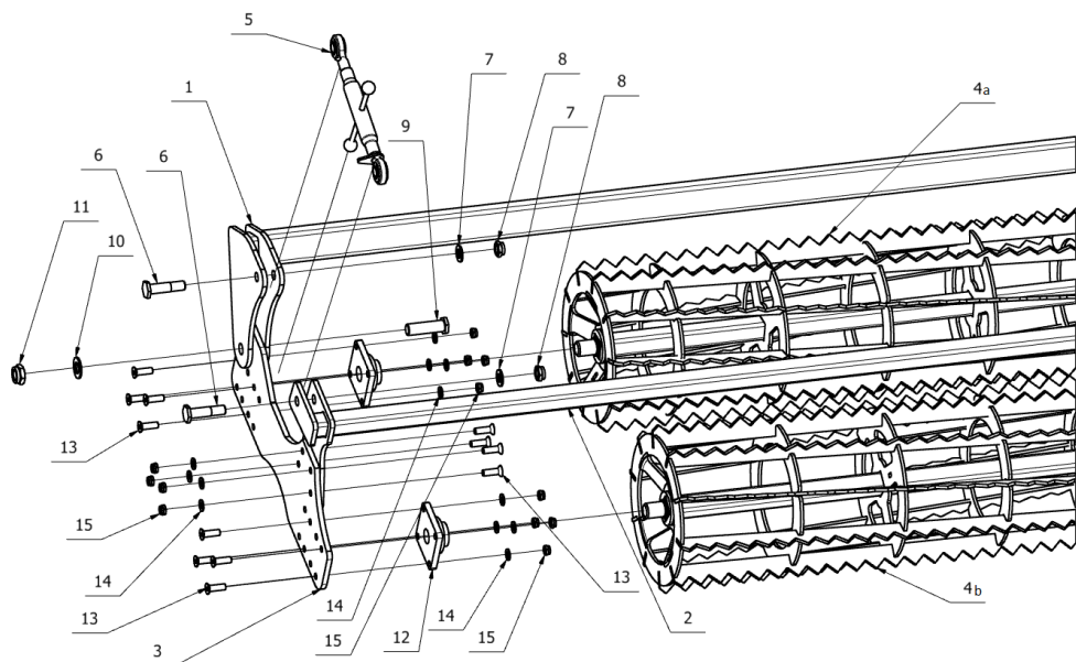
Rys. 61. Wał tandem strunowy Ø420mm.
