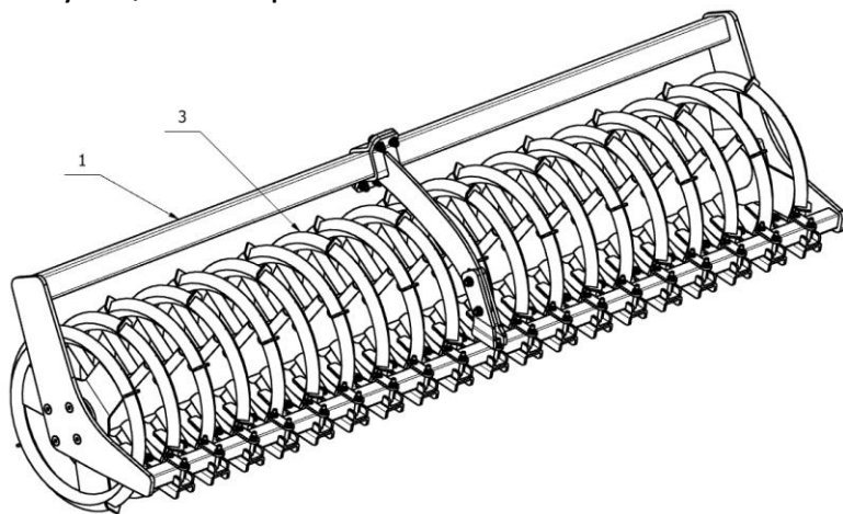
Rys. 29. Wał daszkowy Plus Ø600mm na profilu.
