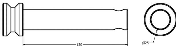
Rys. 71. Sworzeń zaczepowy górny kompletny Ø25mm.
