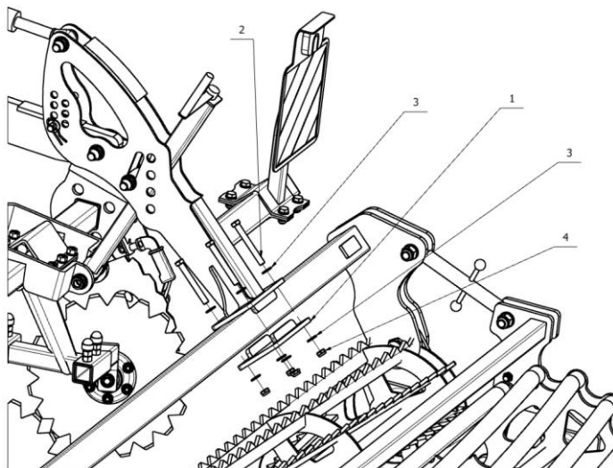
Rys. 14. Mocowanie ramion.
