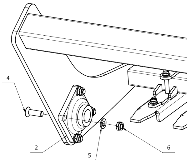
Rys. 38. Wał ceownikowy Ø520mm - mocowanie łożyska.
