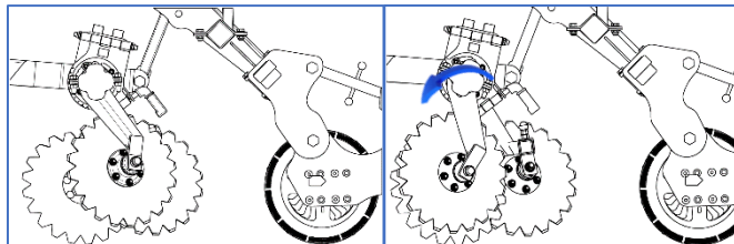
Rysunek 11. Ustawianie głębokości pracy skrajnego talerza.
