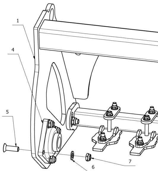
Rys. 48. Wał dyskowy Ø600mm - mocowanie łożyska.
