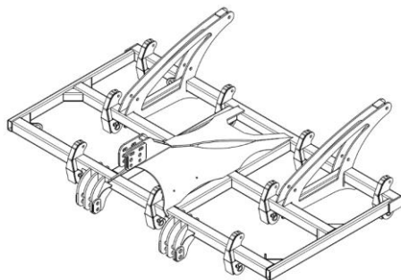
Rys. 1. Rama agregatu z zabezpieczeniem sprężynowym.
